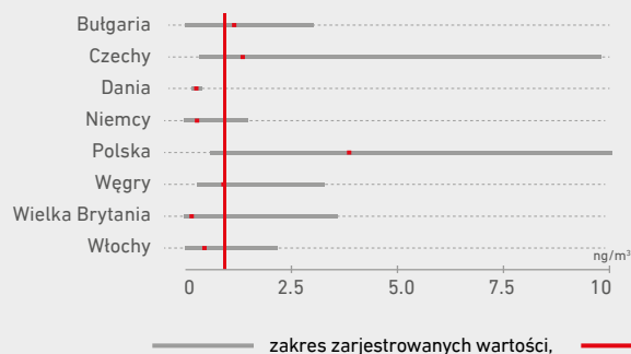
DZIENNA ŚREDNIA KONCENTRACJA ZANIECZYSZCZEŃ BENZO(A)PIRENEM
