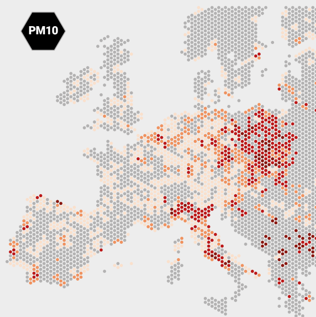
DZIENNA ŚREDNIA KONCENTRACJA ZANIECZYSZCZEŃ PYŁEM PM 10
