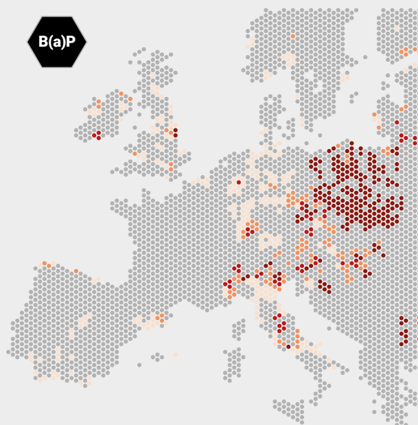
DZIENNA ŚREDNIA KONCENTRACJA ZANIECZYSZCZEŃ BENZO(A)PIRENEM
