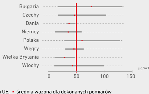
DZIENNA ŚREDNIA KONCENTRACJA ZANIECZYSZCZEŃ PYŁEM PM 10
